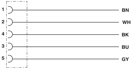
电路图
