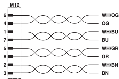
电路图
