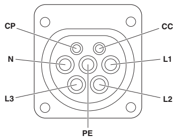
充电装置插座出口的引脚分配
