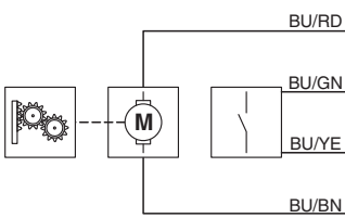
结构框图
