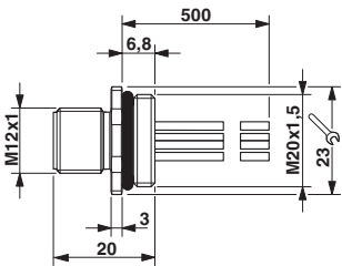
尺寸图
