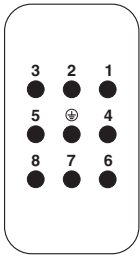
连接器针位分配，连接侧
