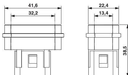
尺寸图
