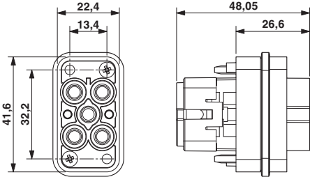
尺寸图
