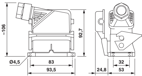
尺寸图
