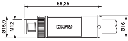
尺寸图
