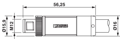
尺寸图
