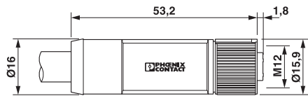
尺寸图
