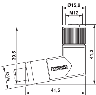
尺寸图
