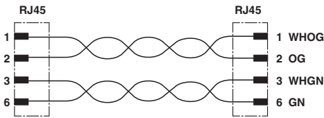
RJ45针式连接器触点分配
