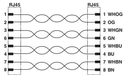
RJ45针式连接器触点分配
