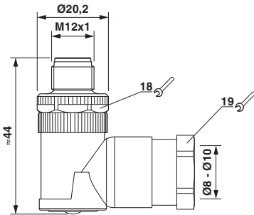
尺寸图
