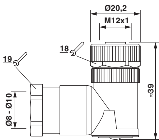
尺寸图
