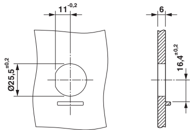
尺寸图
