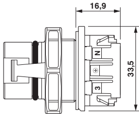
尺寸图
