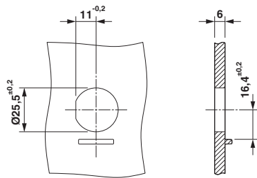
尺寸图
