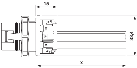
尺寸图
