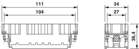
尺寸图
