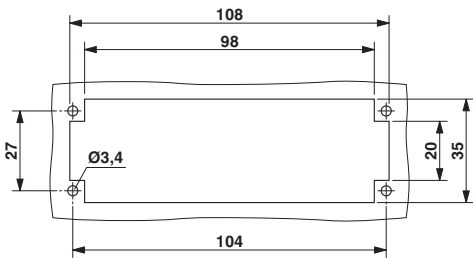
尺寸图
