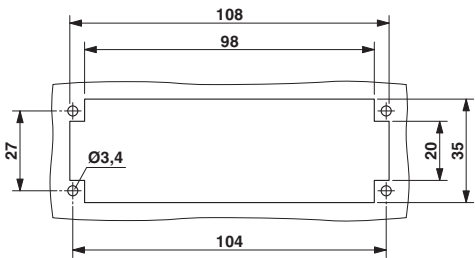
不使用外壳时的安装开口
