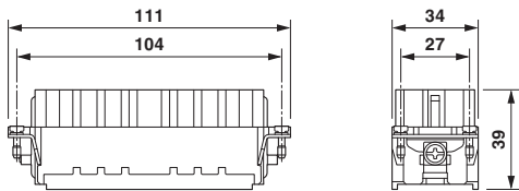
尺寸图
