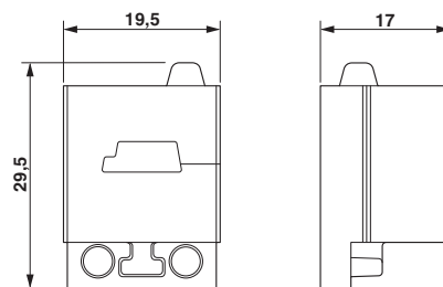
尺寸图
