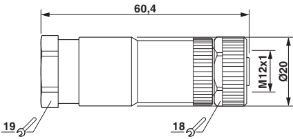
尺寸图
