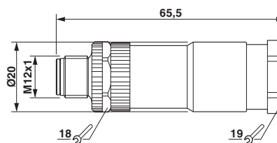
尺寸图
