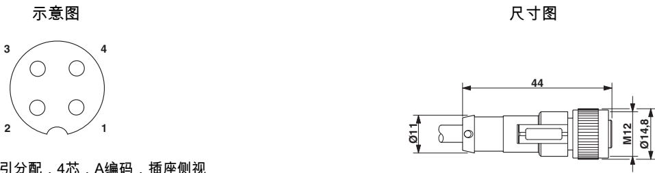
M12孔式连接器引分配，4芯，A编码，插座侧视图
