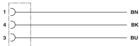
电路图
