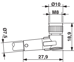
尺寸图
