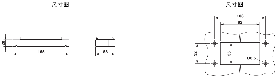
面板开口
