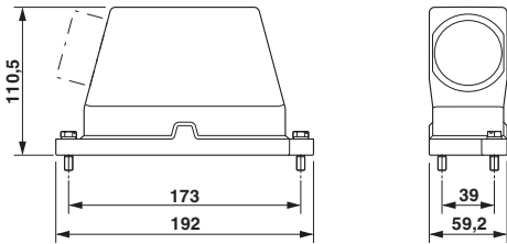
尺寸图
