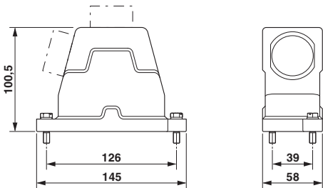
尺寸图
