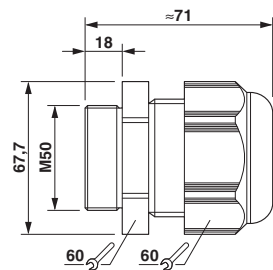
尺寸图
