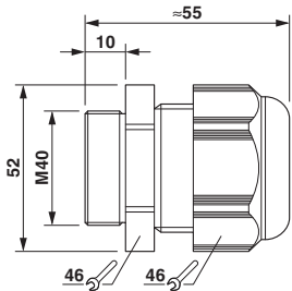
尺寸图
