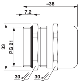
尺寸图
