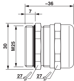
尺寸图
