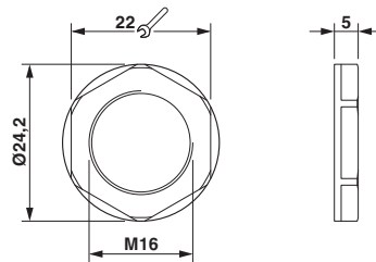
尺寸图
