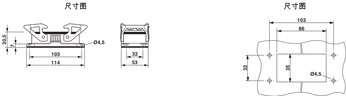
面板开口
