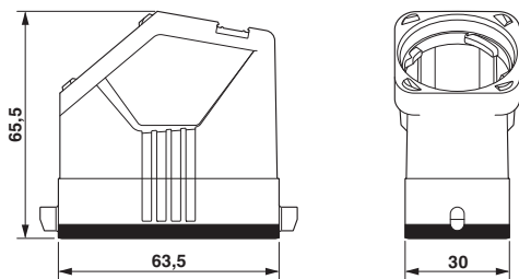
尺寸图
