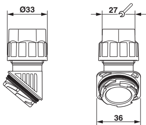
尺寸图
