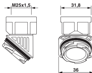
尺寸图
