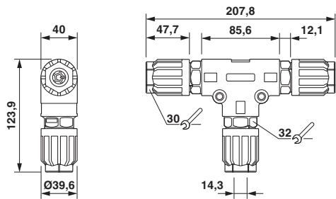
尺寸图
