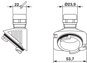
尺寸图
