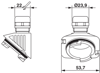
尺寸图
