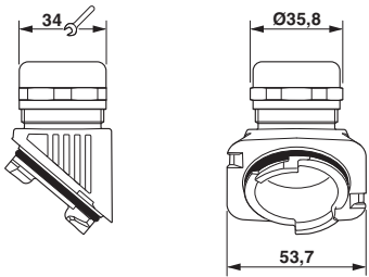
尺寸图
