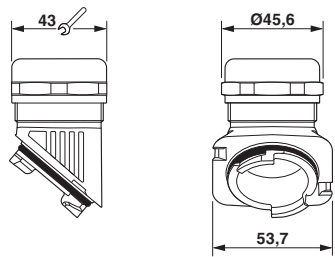
尺寸图
