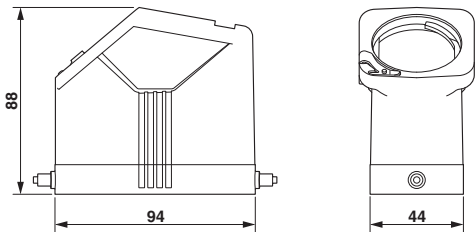
尺寸图
