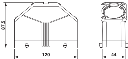
尺寸图
