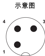
M12针式连接器针脚分配，3芯，A编码，插头侧视图
