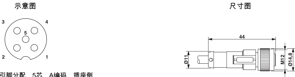
M12孔式连接器引脚分配，5芯，A编码，插座侧视图
