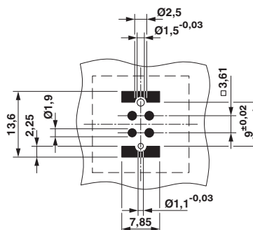
钻孔图
