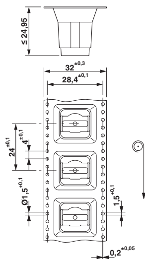
尺寸图
