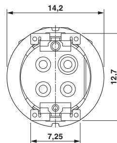
尺寸图
