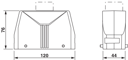
尺寸图
