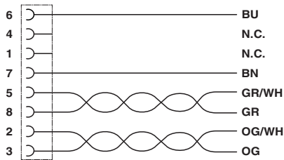
电路图
