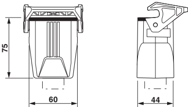
尺寸图
